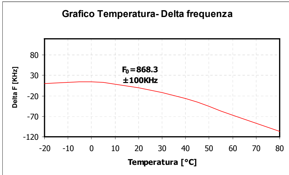
Fig. 6 Andamento del delta frequenza in funzione della temperatura.
