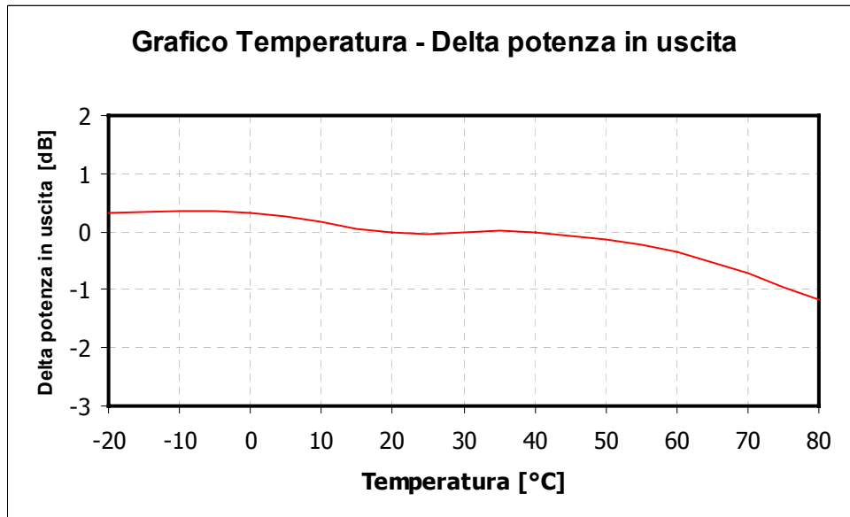
Fig. 4 Andamento del delta potenza RF in funzione della temperatura.
