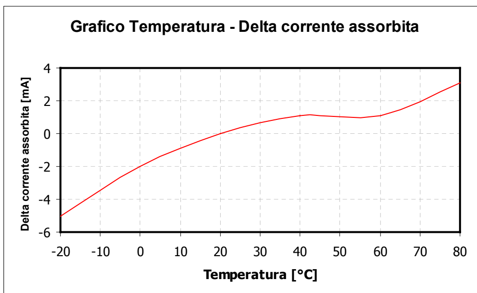
Fig. 5 Andamento del delta corrente assorbita in funzione della temperatura.
