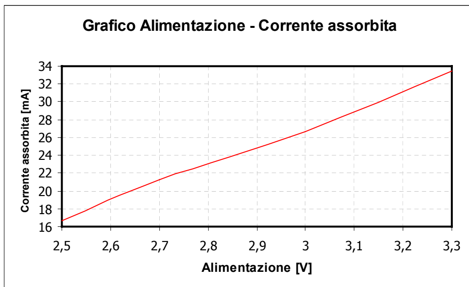
Fig. 3 Andamento della corrente assorbita in funzione della tensione di alimentazione.
