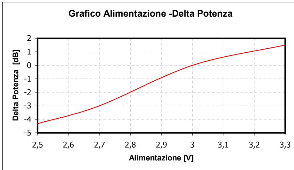
Fig.2 Andamento del delta potenza RF in funzione della tensione di alimentazione.
