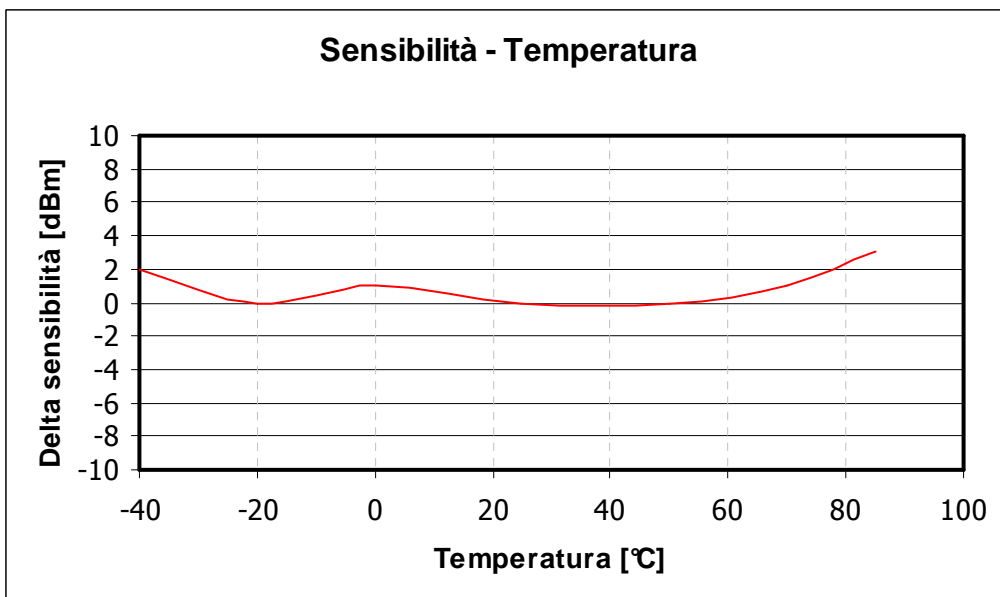
Fig. 5 – Delta sensibilità in funzione della temperatura
