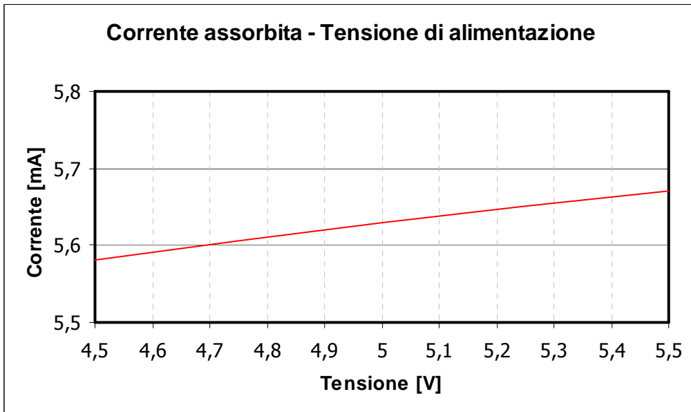
Fig. 4 – Andamento corrente in funzione della tensione
