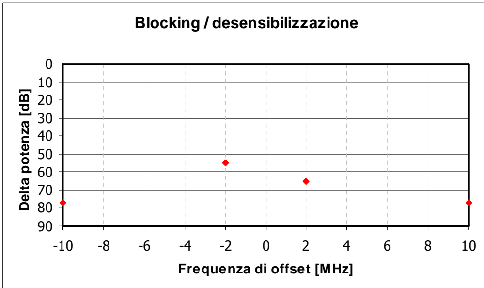
Fig. 6 – Misura di blocking secondo la Normativa ETSI EN 300 220-1
