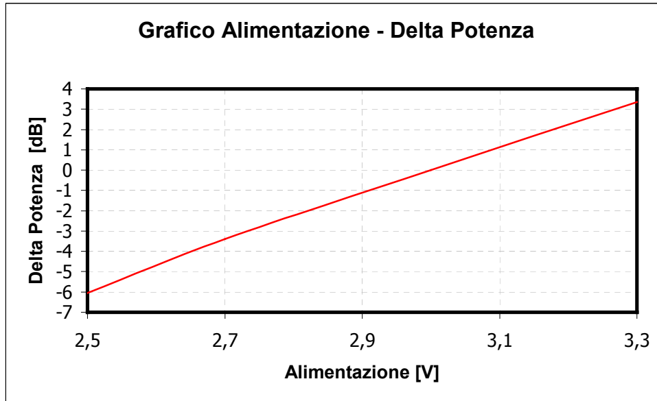
Fig. 3 Andamento del delta potenza RF in funzione della tensione di alimentazione
