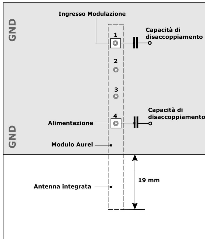
Fig. 1: lay-out consigliato per un corretto funzionamento del dispositivo
